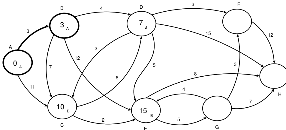
Figura 8.11: Aggiornamento dei pesi partendo da B
