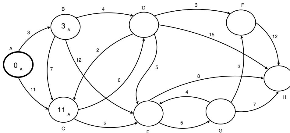
Figura 8.10: Aggiornamento dei pesi partendo da A
