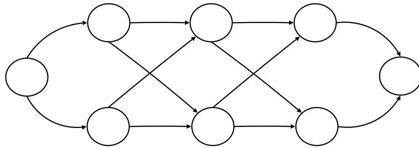
Figura 8.8: Cammini possibili
