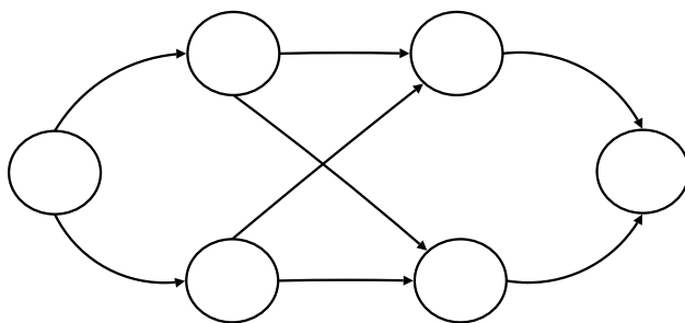
Figura 8.7: Cammini possibili
